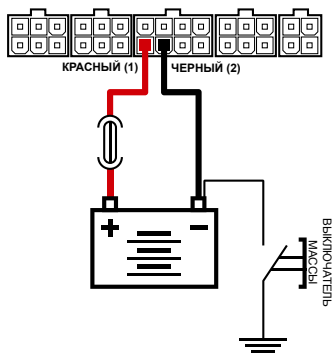
Подключение питания до выключателя массы
